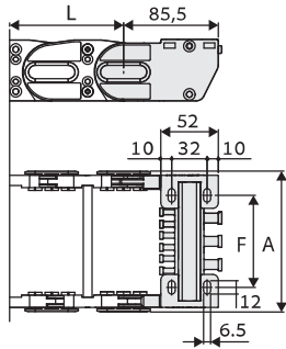
קצוות מניילון - סוג 1
