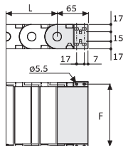
קצוות מניילון - סוג 1
