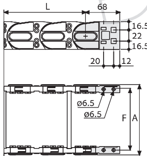
קצוות מניילון - סוג 2
