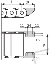
קצוות מניילון - סוג 2
