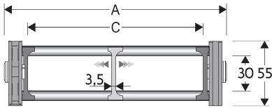
קצוות מניילון - סוג 1
